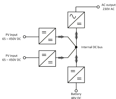
Convertisseur solaire RS Smart 48/6000
